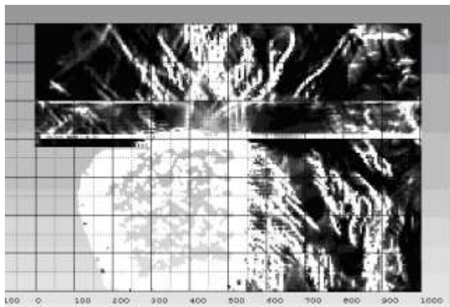
Рисунок 4 - Процесс трещинообразования в углепородном массиве в окрестности взрыва зарядов ВВ в призабойной части выработки, t = 12 мс
